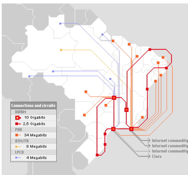
Figura 1: la dorsale di Brasil Telecom
